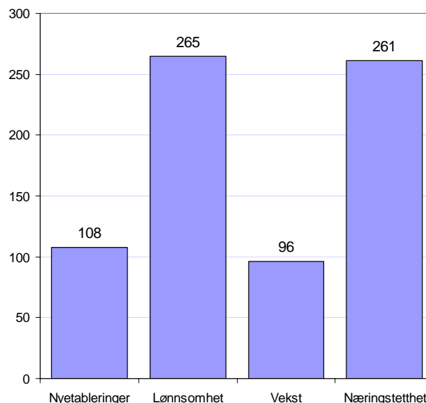
Figur 25: Giskes rangering for de ulike delindeksene som inngår i næringslivsindeksen, 2006.
