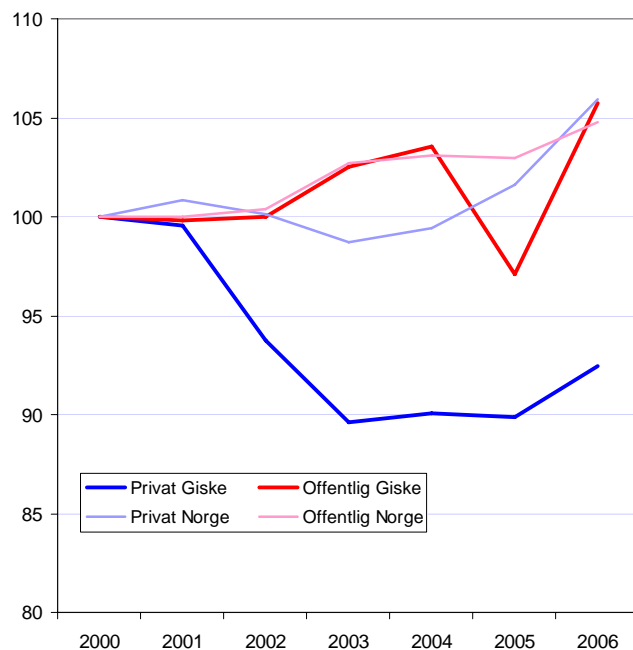
Figur 8: Utvikling i antall sysselsatte, privat og offentlig i Giske og Norge.
