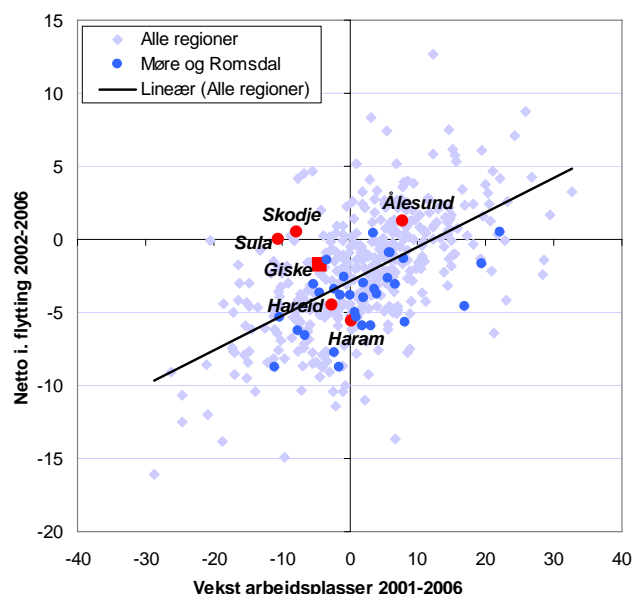
Figur 13: Sammenhengen mellom nettoflytting og endring i arbeidsplasser i kommuner i Norge og Møre og Romsdal.
