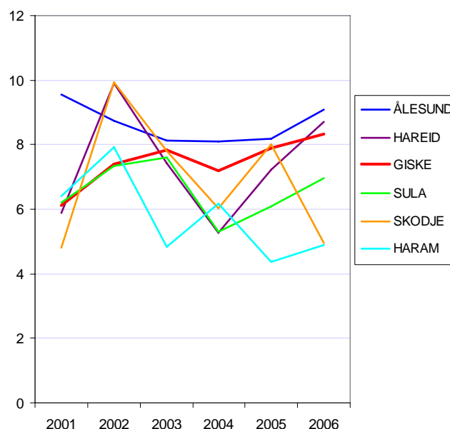
Figur 22: Etableringsfrekvens i Giske og nabokommuner.
