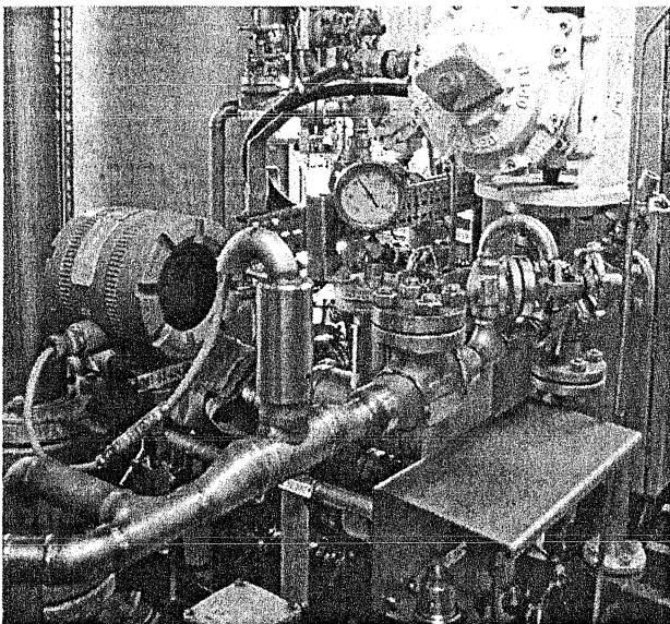
Figur 6.7: En konduktivitetmåler sørger for at produsert vann automatisk sjekkes, og dumpes dersom grensen på 6 mS/m overskrides (Foto: Eyvind Andersen)
