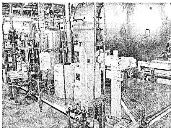
Figur 1.1: Drikkevannsanlegg med evaporator, avleiringshemmertank, klortank, alkaliseringsfilter og UV-anlegg (Foto: Eyvind Andersen)
