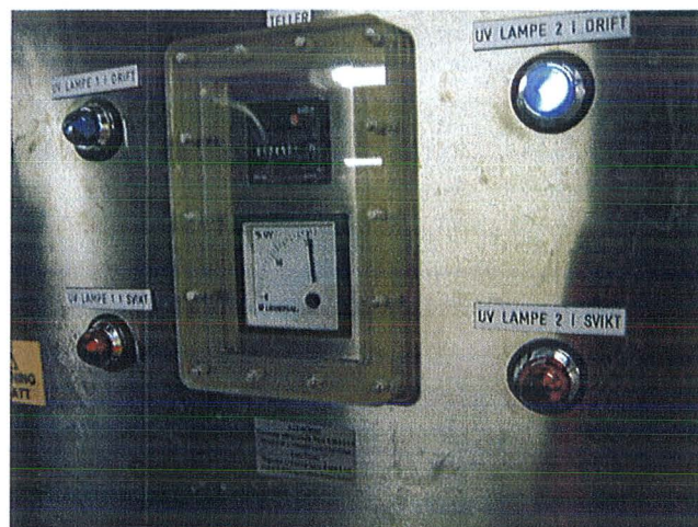
Figur 8.6: Kontrollpanel for UV-anlegg med to UV-strålerør. Blått lys viser at strålerør nummer to er i drift og fungerer. Midt på bildet skimtes timeteller (sort) og UV-intensitetsmålerskive (Foto: Eyvind Andersen)
