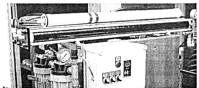
Figur 6.6: Omvendt osmoseanlegg. Membranen er en rull inne i røret øverst (Foto: Bjørn Løfsgaard)
