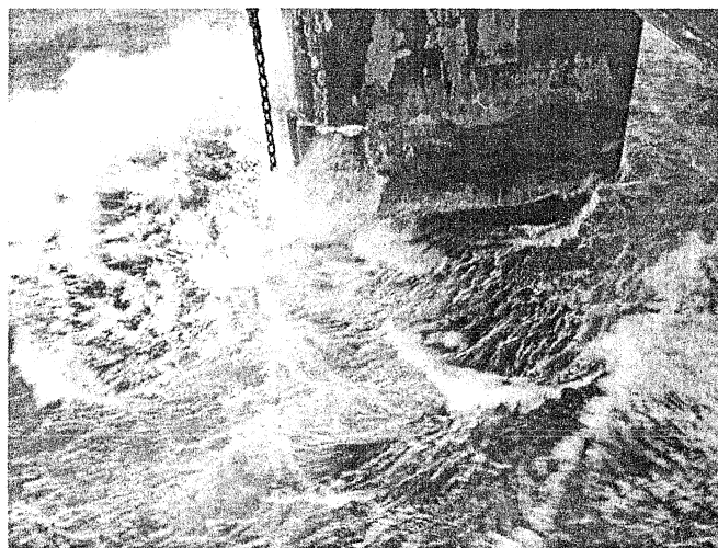
Figur 6.1: I området rundt plattformbeina er det stor turbulens, og sjøvannsinntakene må plasseres der hvor risikoen for forurensning er minst (Foto: Eyvind Andersen)
