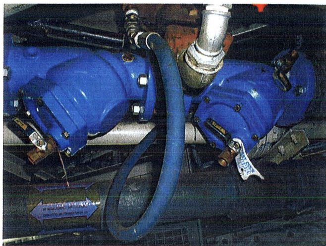
Figur 9.5: Andre væskesystemer bør ikke forsynes med drikkevann. Der dette ikke kan unngås, gir brutt forbindelse eller doble tilbakeslagsventiler med drenering imellom (bildet) best sikring (Foto: Eyvind Andersen)
