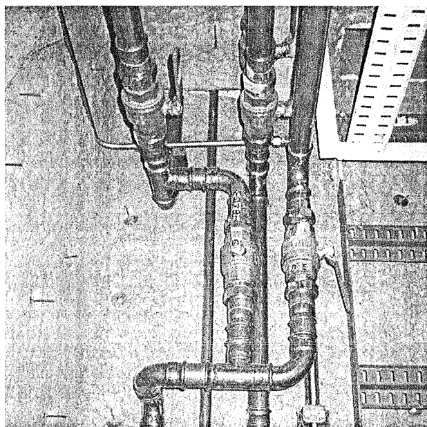
Figur 4.7: Korrosivt vann i kopperrør kan føre til for høye kopperverdier i drikkevannet (Foto: Bjørn Løfsgaard)
