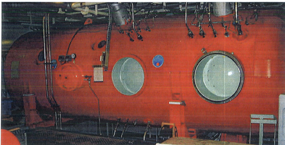
Figur 10.1: Trykkammer for dykkeroperasjoner (Foto: Eyvind Andersen)
