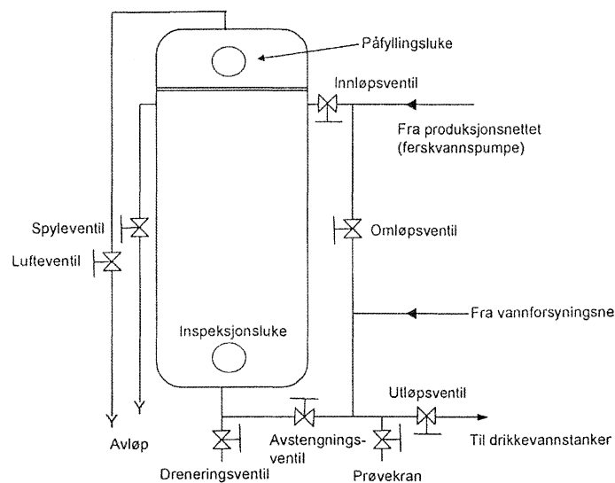
Figur 8.1: Filteret må bygges slik at det er lett å komme til ved rengjøring, utskifting av masse og annet vedlikehold (Ill.: Karin Melsom)
