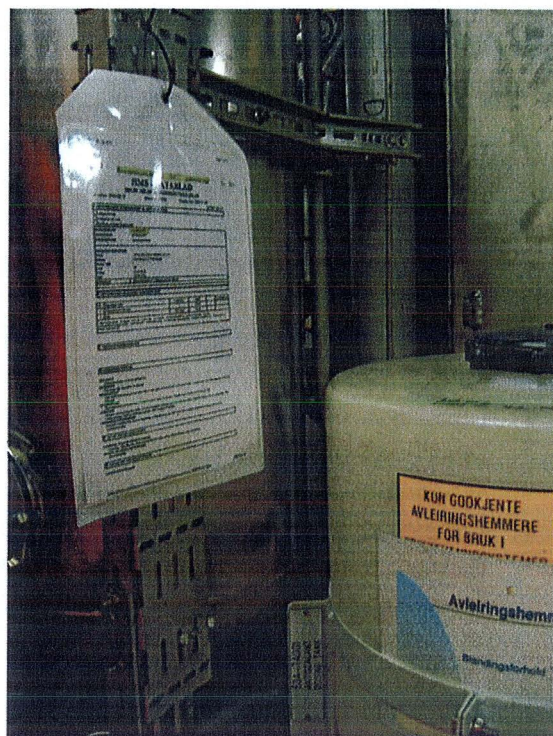
Figur 5.3: Godt merket og sikret tank for avleiringshemmer (Foto: Eyvind Andersen)
