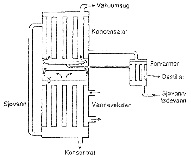
Figur 6.3: Prinsippskisse for vakuumbestillering (Ill. hentet fra B3/NIVAs tegnekontor)
