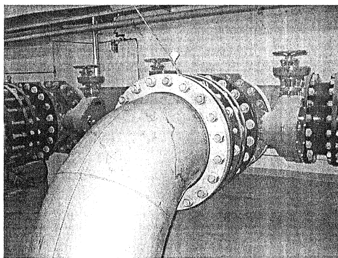
Figur 9.6: Rør og ventiler i drikkevannssystemer finnes i mange forskjellige størrelser og materialer. Man bør velge materialer som er korrosjonsbestandige, og som ikke gir opphav til biologisk vekst (Foto: Eyvind Andersen)
