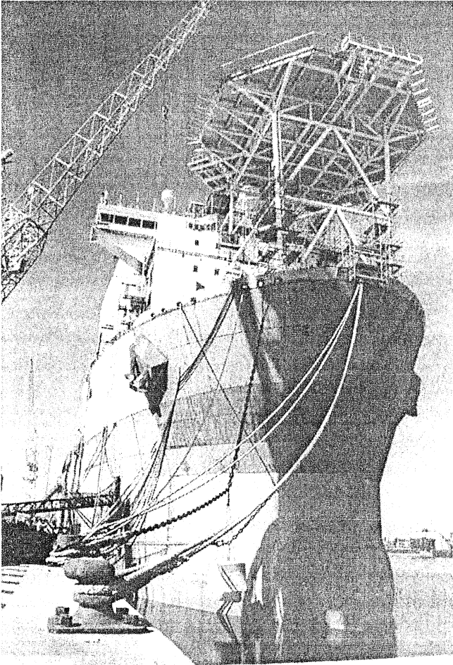
Figur 2.1: Bilde av innretningen Navion Odin, tatt på verftet (Foto: Eyvind Andersen)
