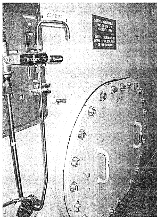
Figur 9.3: Bildet viser lett tilgjengelig prøvetakingskran og mannhull for drikkevannstank (Foto: Eyvind Andersen)
